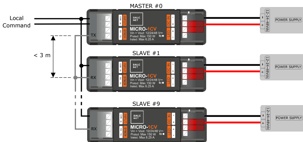
Figura 8: Schema di collegamento del segnale Sync con un alimentatore per ogni dimmer
