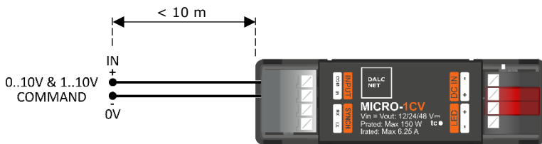
Figura 5: Schema di collegamento dei segnali analogici 0-10V e 1-10V
