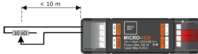
Figura 6. Il rilevamento automatico del potenziometro parte con un valore compreso tra il 30% e il 70%.
