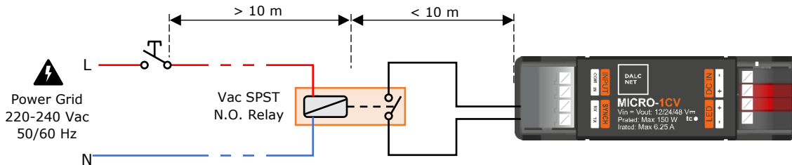
Figura 4 mostra un esempio di schema elettrico di comando locale consigliato per lunghe distanze. Si noti che questo diagramma funziona solo per l'input tramite pulsante.
