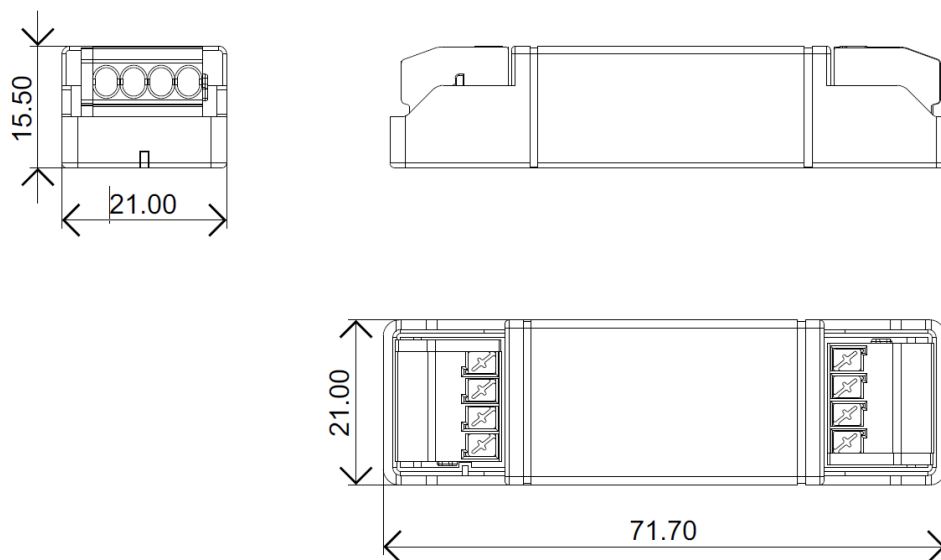
Figura 12: Dimensioni meccaniche
