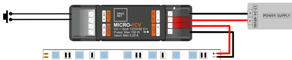
Figura 2: Schema di collegamento dei carichi LED bianchi o monocolore
