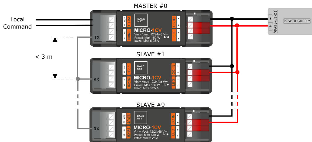
Figura 7: Schema di collegamento del segnale Sync con un singolo alimentatore
