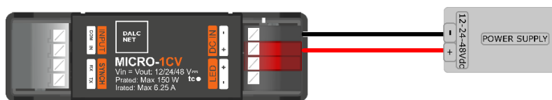
Figura 9: Schema di collegamento dell'alimentatore
