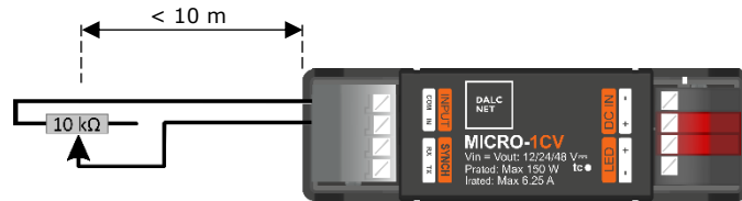
Figura 6: Schema di collegamento del potenziometro
